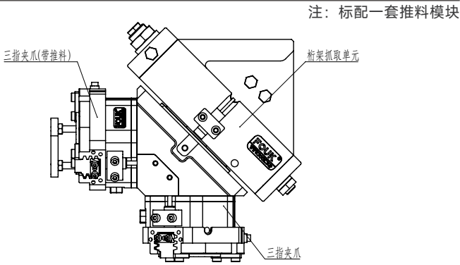
注：连接板根据不同需求设计不同厚度 A; 标配一套推料模块
