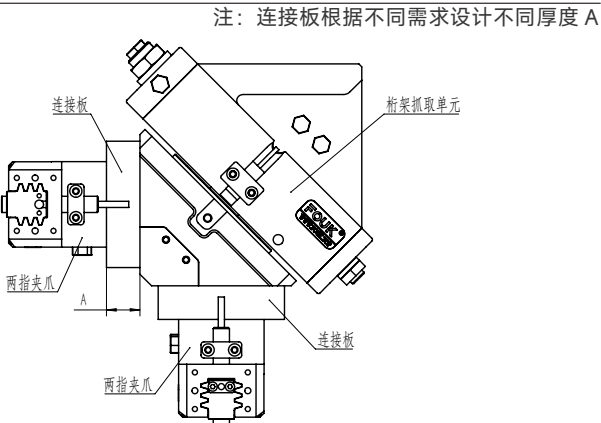
注：连接板根据不同需求设计不同厚度 A
