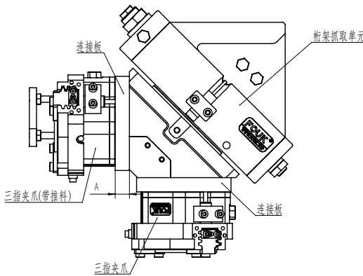
注：连接板根据不同需求设计不同厚度 A; 标配一套推料模块
