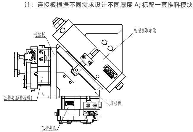
注：连接板根据不同需求设计不同厚度 A
